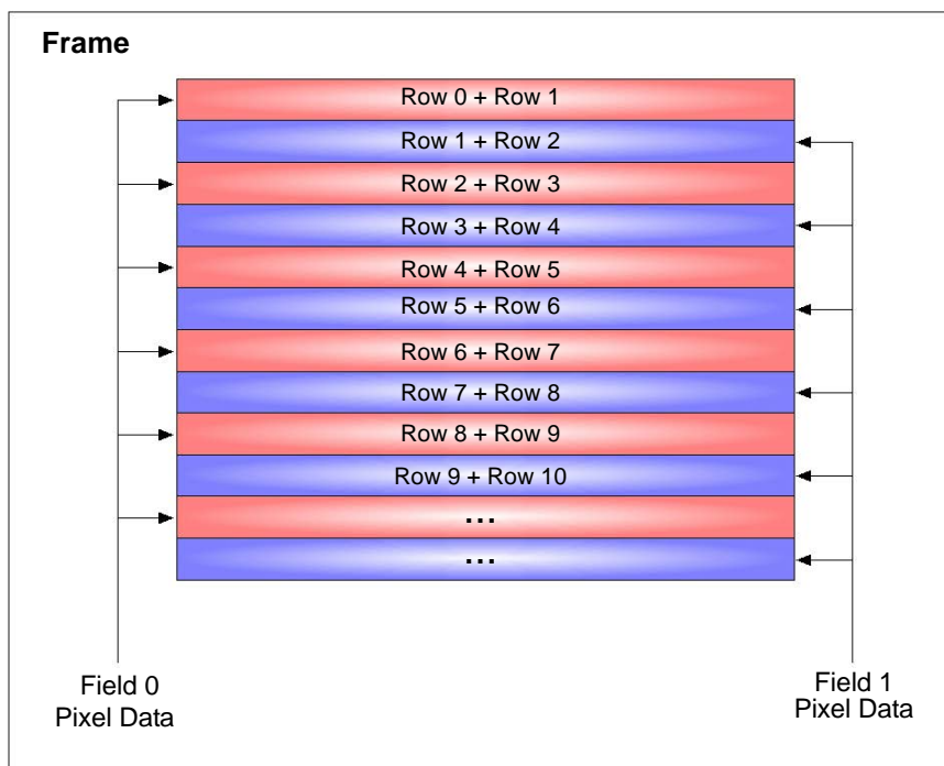
Fig. 60: Deinterlaced New Fields Output Mode
