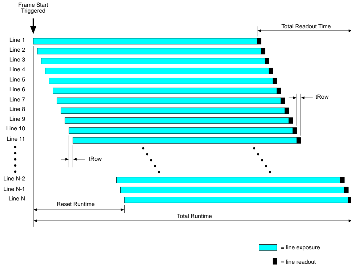
Fig. 62: Rolling Shutter in the ERS Mode
