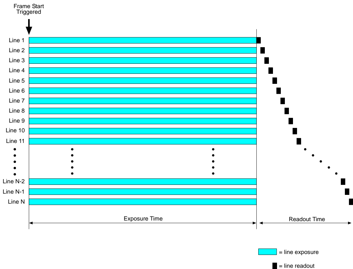
Fig. 61: Global Shutter
