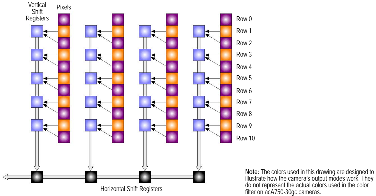
Fig. 56: Field 1 Readout
