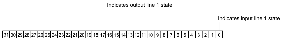
Fig. 123: Line Status All Parameter Bits
